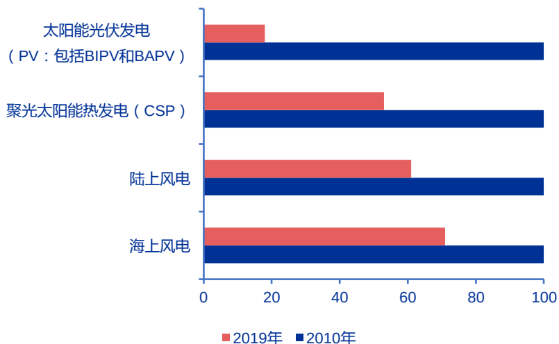
光伏发电成本降幅最大（单位：%）
