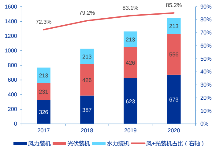
公司发电装机构成以风光为主（单位：MW）
