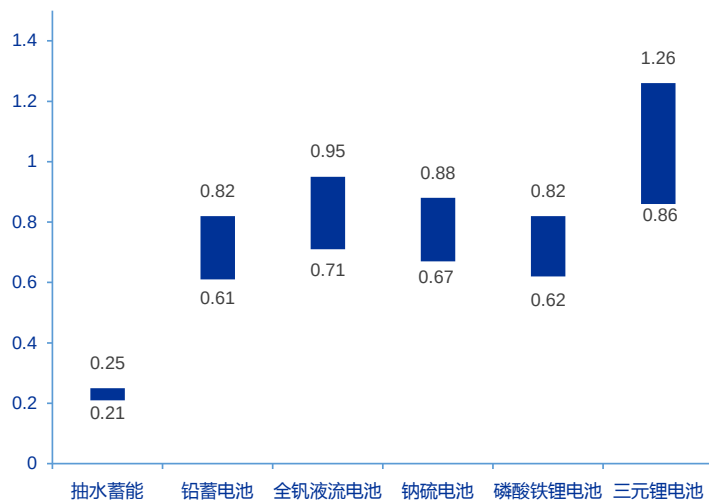
抽水蓄能经济性远高于电化学储能（单位：元/KW.h）
