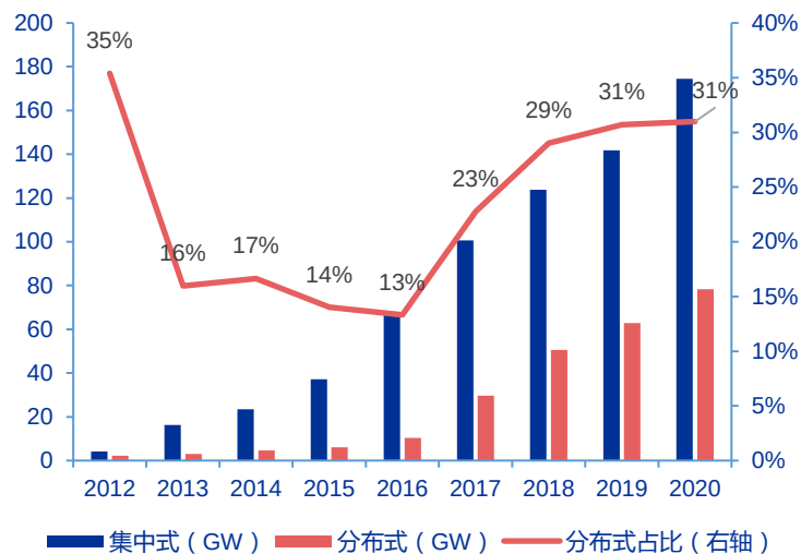
近四年分布式光伏增速CAGR为66%
