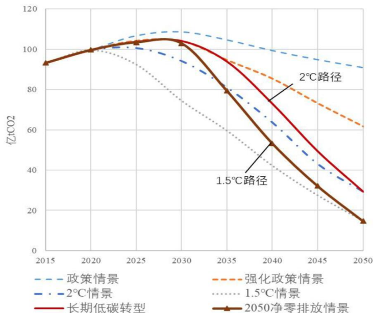
不同减排力度下我国二氧化碳排放量预测
