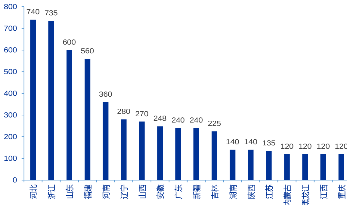
在建抽蓄电站装机容量以河北和浙江最多（单位：万千瓦）
