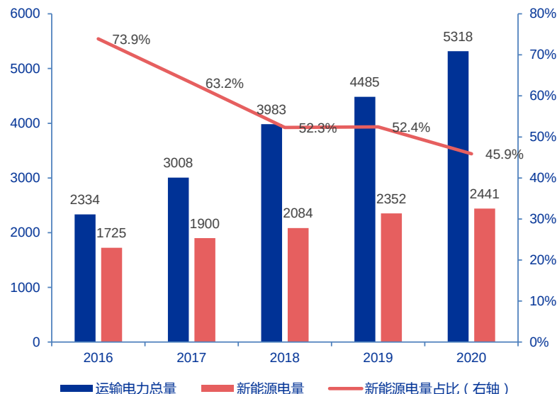
2020年特高压输送电量中新能源电量占比45.9% (单位：亿千瓦时)
