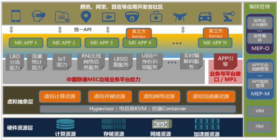
图 39: 中国联通边缘业务平台架构图
