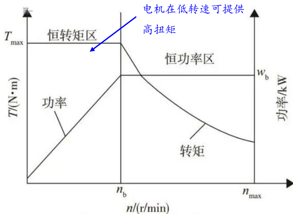
图表：驱动电机扭矩特性图
