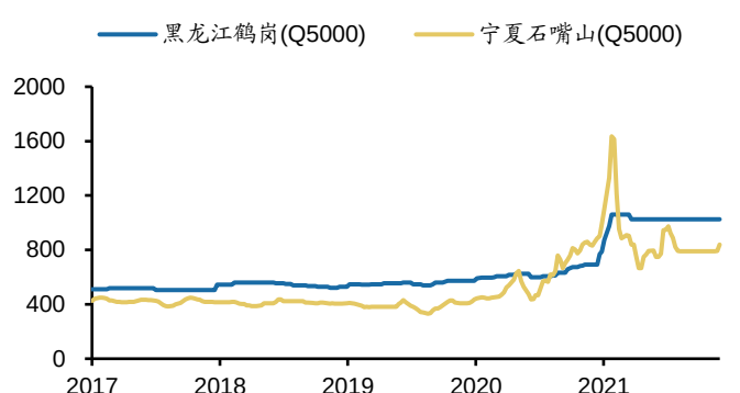
图 31：其他地区动力煤车板价（元/吨）
