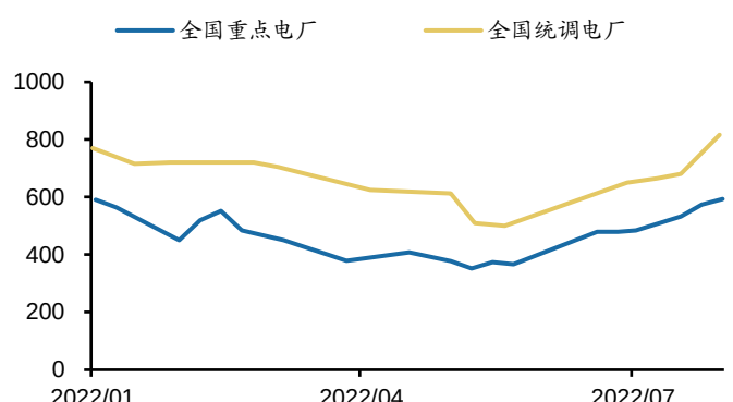
图 33：全国电厂日耗煤炭情况（万吨）
