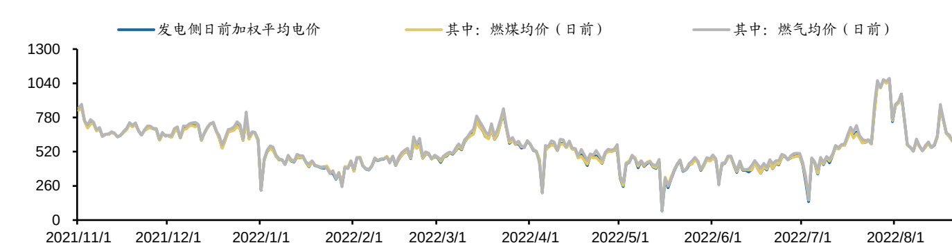
图 36: 广东电力交易中心现货日前交易情况（单位：元/兆瓦时）
