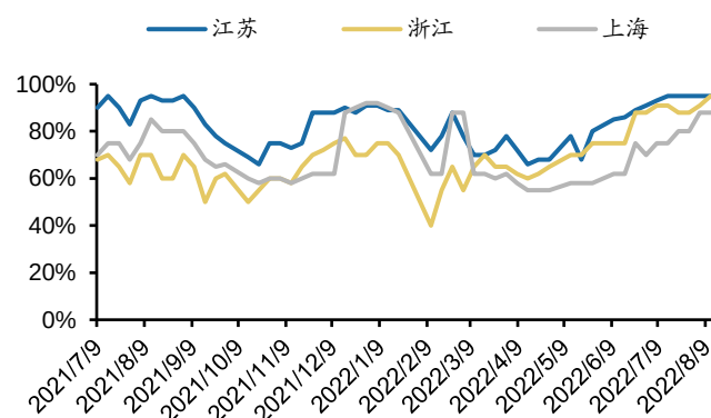
图 37: 江浙沪地区电厂负荷率波动情况
