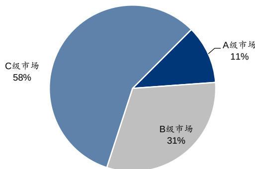
图表26：2020年欧派家居门店分布（按市场级别，单位：家）
