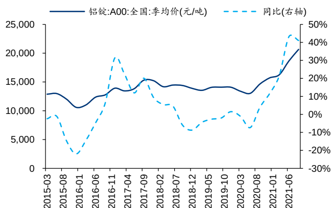
图表80： 2015年以来铝锭价格情况
