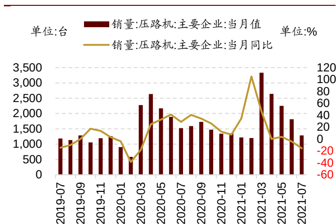
图 15: 7 月主要企业压路机销量同比下降 15.50%
