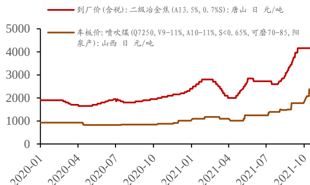
图 2：2020 年至今煤炭价格变化情况
