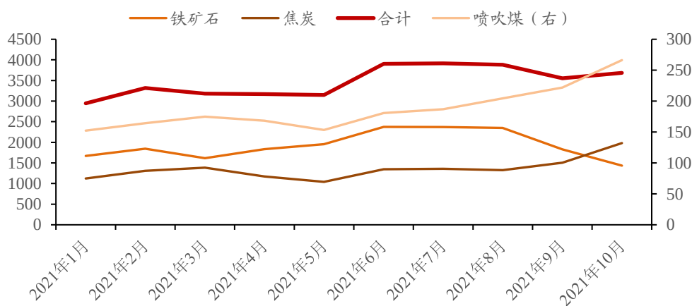
图 3：2021 年单月吨钢原料成本测算（成本滞后一个月；元/吨）
