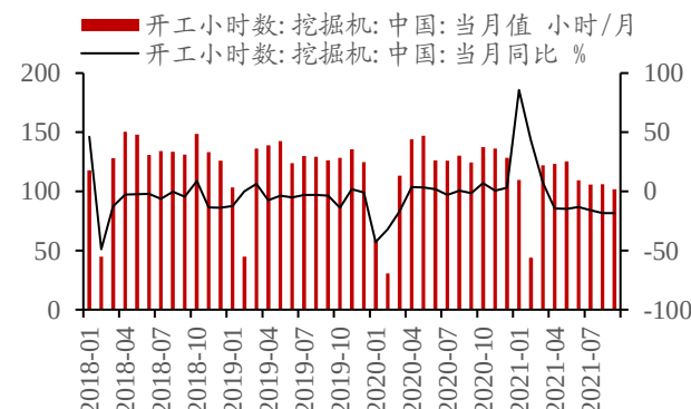
图 12：挖掘机开工小时数
