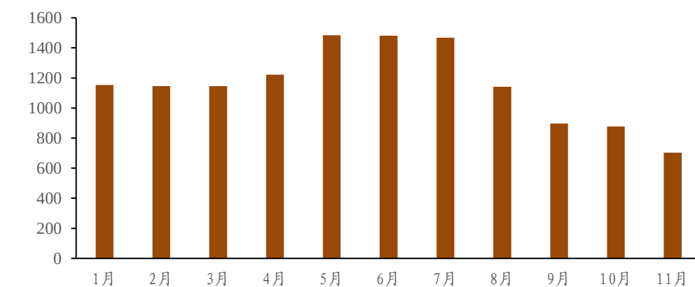
图 15：2021 年铁矿石现货价格指数(CSI):进口粉矿:62%Fe 月度均价（元/湿吨）
