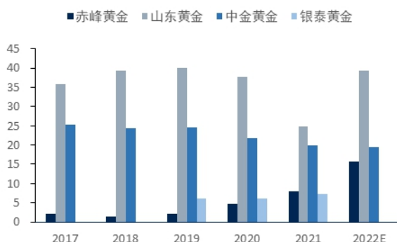
图42: 分公司金产量变化 (吨)
