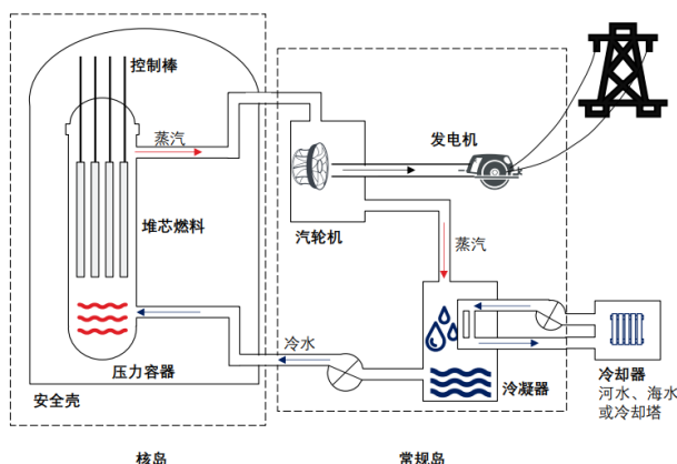
图 23：通用核电站工作流程
