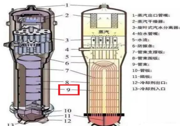
图 24：核电蒸发器及 U 形管示意图
