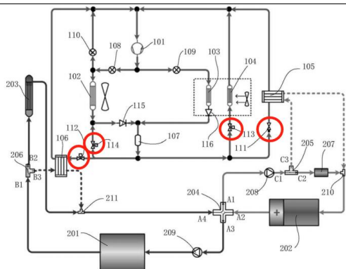
图 4：蔚来热泵空调系统的一种解决方案中包含 4 个电子膨胀阀
