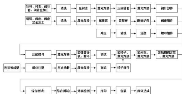
图 13：空调电子膨胀阀的生产工艺
