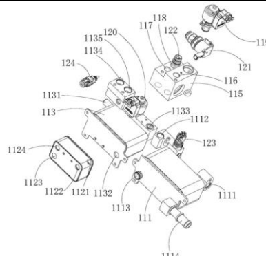
图 12：小鹏专利中提及的热管理集成单元阀、换热类相关部件拆解
