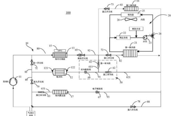
图 9：比亚迪专利中提及双向膨胀组件（图中虚线框内）
