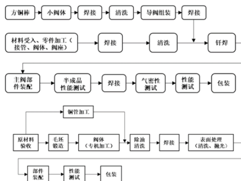
图 14：空调四通阀（上图）、截止阀（下图）的生产工艺
