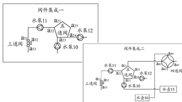
图 10：华为专利中提及阀件总成
