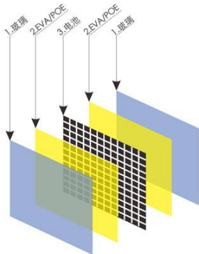
图 38、双玻组件结构图
