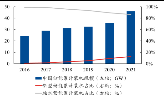
图 10、国内新型储能占比快速增长
