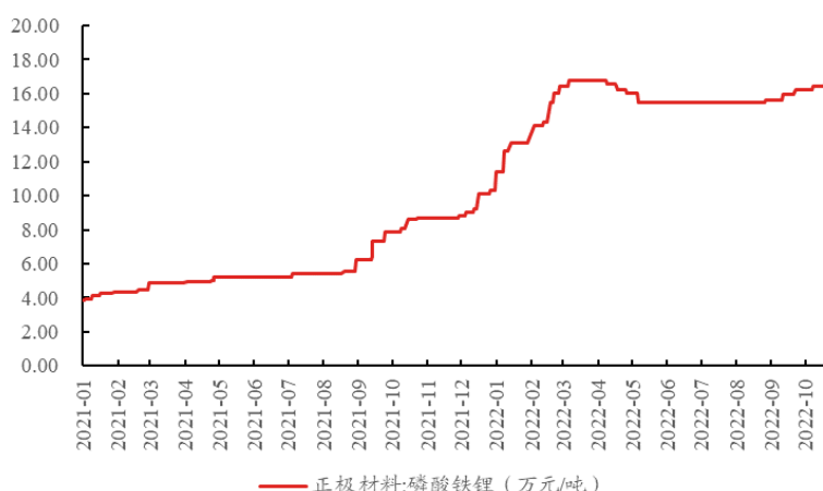
图 13、2022 年磷酸铁锂正极材料价格上涨
