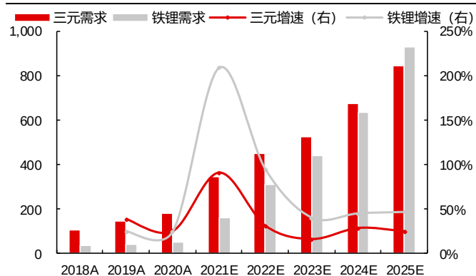
图 13: 全球三元与磷酸铁锂电池的需求及增速估算 (GWh)
