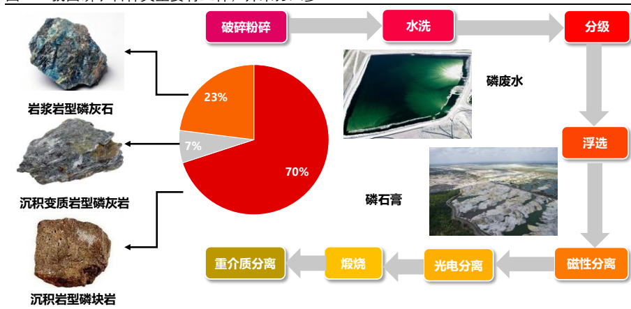
图 1: 我国磷矿石种类主要有三种, 开采分八步
