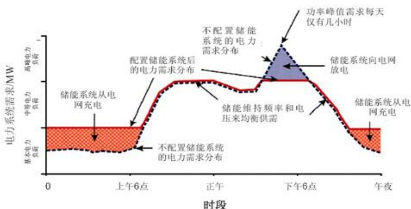
图 57：储能系统在电网中的削峰填谷作用
