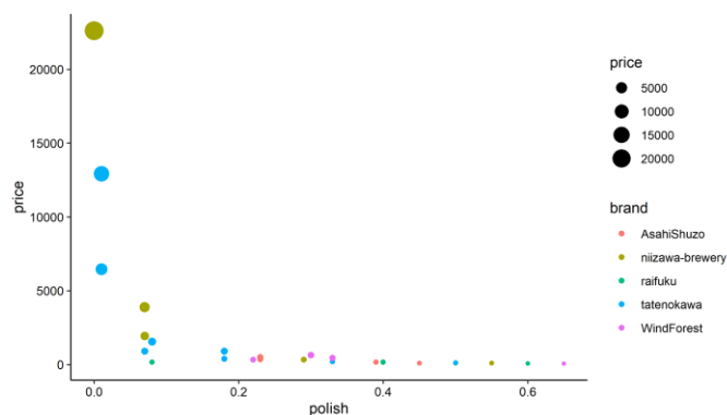
图 24：清酒价格与精米步合呈负相关关系
