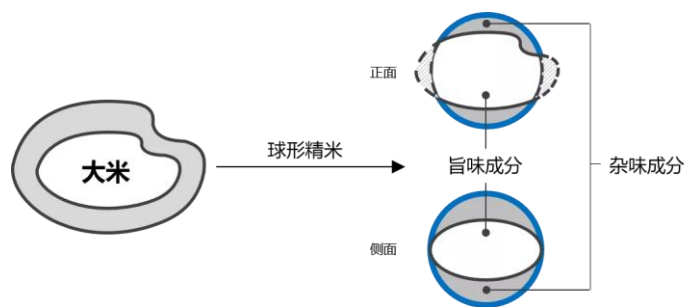
图 25：精米旨味及杂味成分
