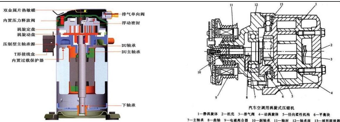
图表 36：空调压缩机（左）与汽车空调压缩机（右）具有接近的底层原理
