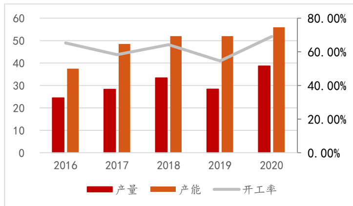
图26 国内PA66生产情况（万吨；%）
