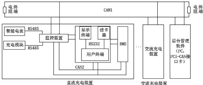
图6 充电站系统框图
