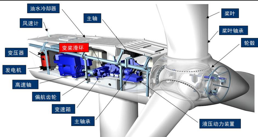
图8 典型风轮结构图
