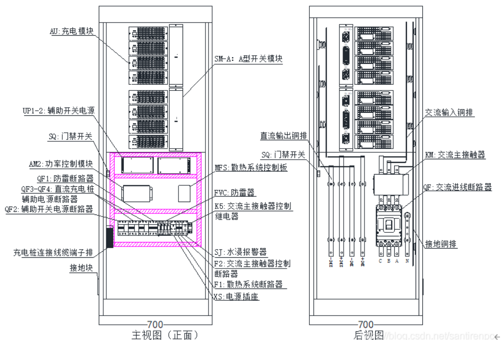
图5 160kW 分体式双充接口充电柜内部元器件布置
