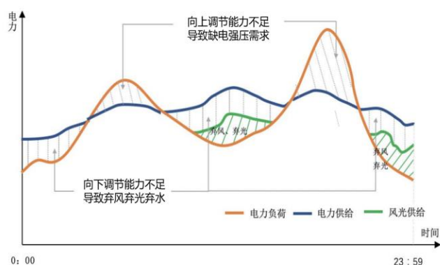
图 23：电力系统向上与向下灵活性不足原理
