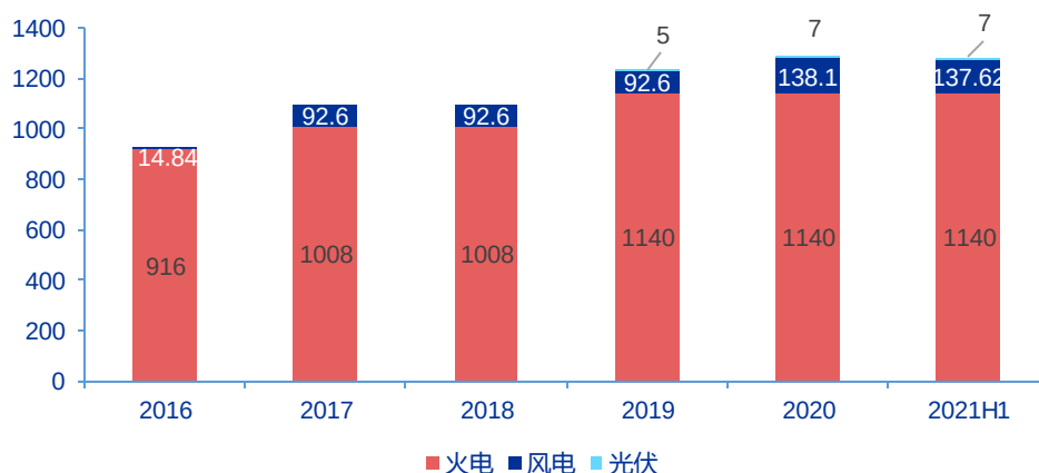
图 2：2016-2021H1 公司装机量变化情况（万千瓦）
