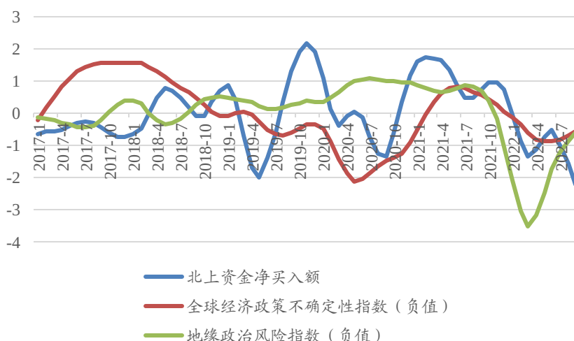
图 4 北上资金流向与全球风险水平的关系（经去噪、标准化）
