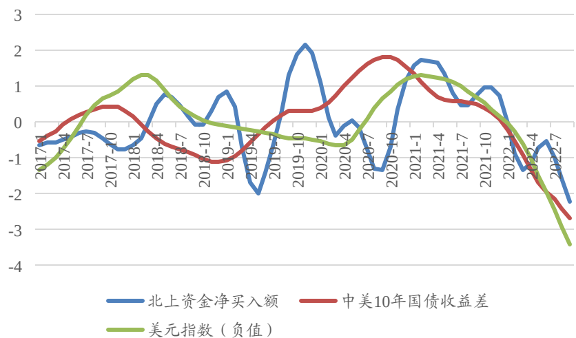
图 3 北上资金流向与利率汇率之间的关系（经去噪、标准化）
