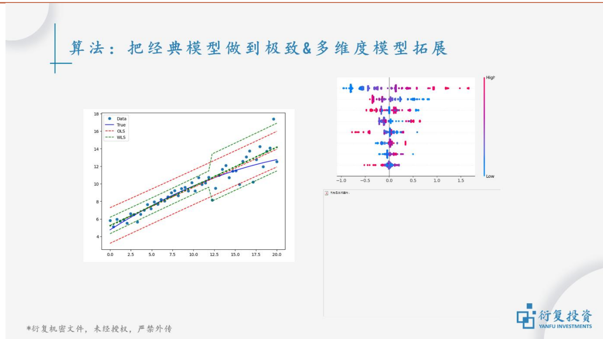
图 32 算法比较
