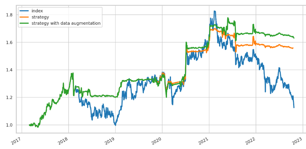
图 35：策略净值对比（预测器：Logistic regression）
