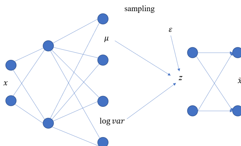
图 4: VAE 架构示意图
