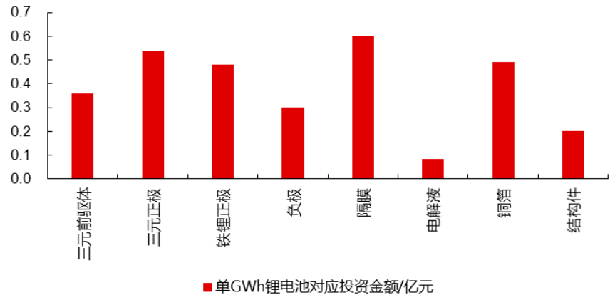
图 25：铜箔单 GWh 锂电池对应产能的投资金额较高
