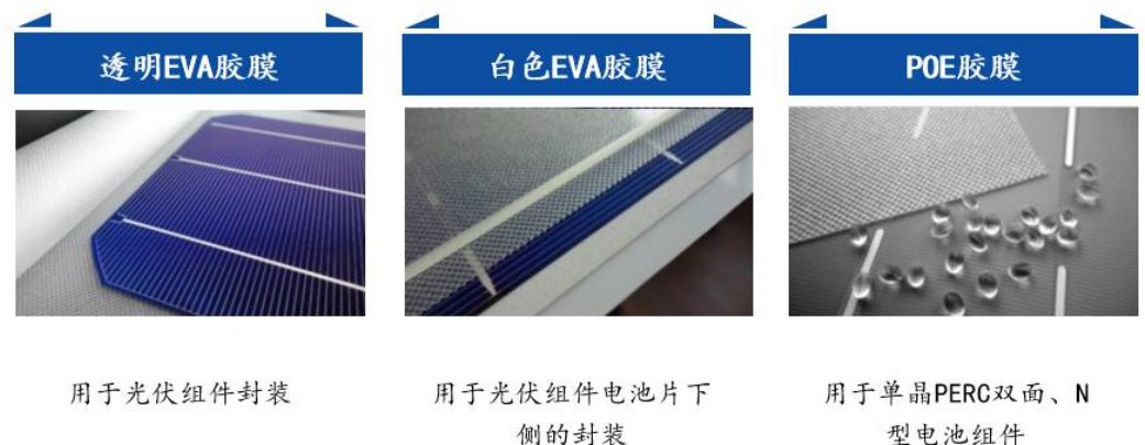
图表 17 光伏胶膜的产品类别
