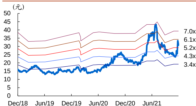
图 34: 莱克电气历史 PB Band
