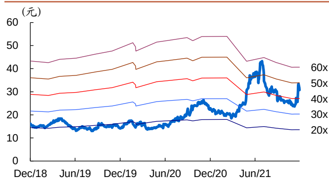
图 33: 莱克电气历史 PE Band
