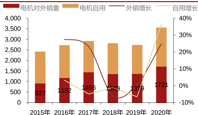
图 4：莱克电机一半对外销售（万台/%)
