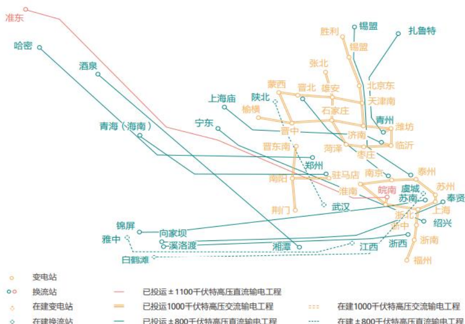
图 9：国家电网的跨区域特高压输电通道
