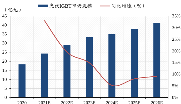
图 67: 2026 年我国车规级 IGBT 规模有望达 22.3 亿美 图 68: 2026 年我国光伏用 IGBT 规模有望超 40 亿
