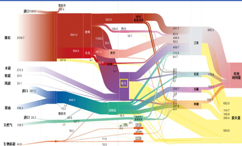
图 1：我国能流图示意（百万吨标煤，数据为 2012 年，我国当前新能源占比更高，但是基本结构变化不大）
