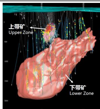
图9 丘卡卢-佩吉上矿带顶部存在超高品位分布集中矿体
