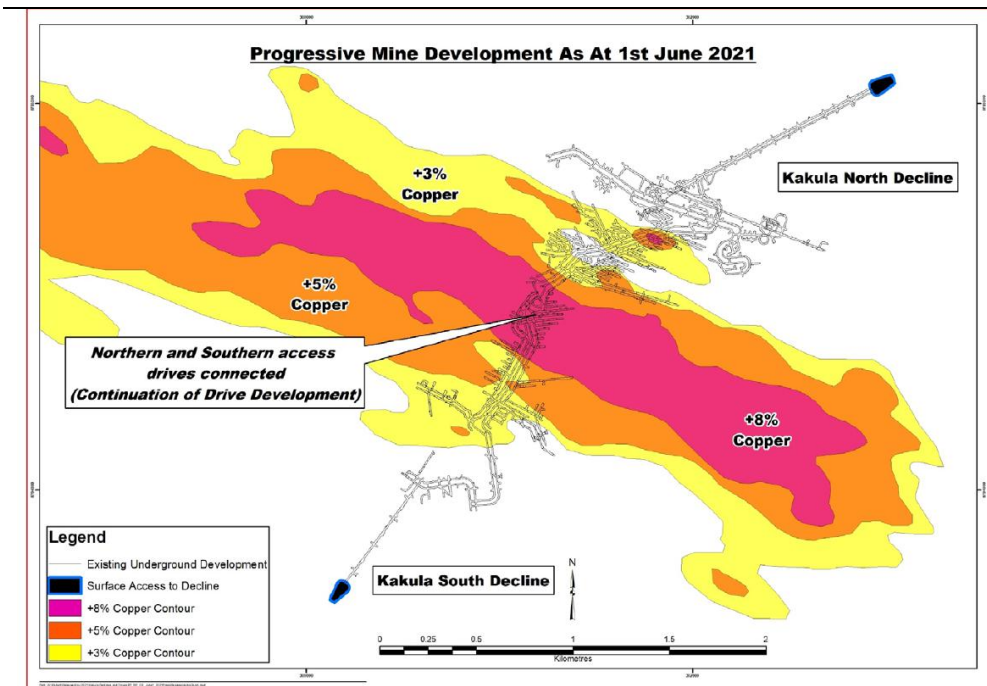
图3 卡莫阿-卡库拉矿区中心玫红色为品位高达 8%的铜矿
