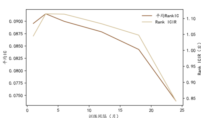
图 7：不同训练频率的累积平均 RankIC 和 Rank ICIR
