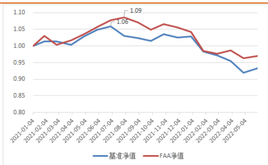
图 1、基准策略和 FAA 策略的净值曲线
