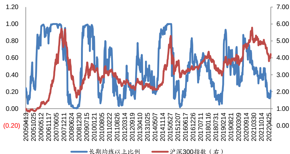
图12: 市场情绪之200日长期均线之上比例数据
