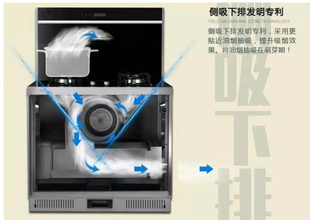
图 4：侧吸下排技术工作原理示意图
