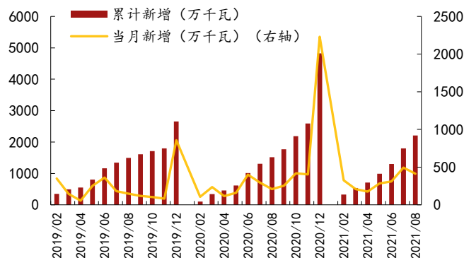
图 80: 近年光伏装机量稳步上涨
