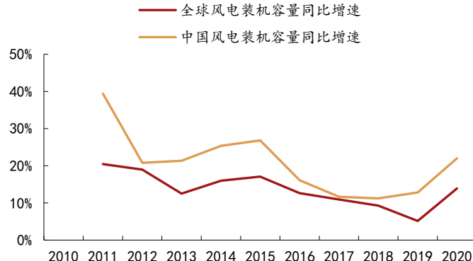
图 91：中国风电装机容量增速高于全球
