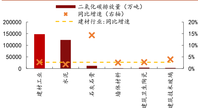
图 58：2020 年建材各子行业碳排放量均同比增长
