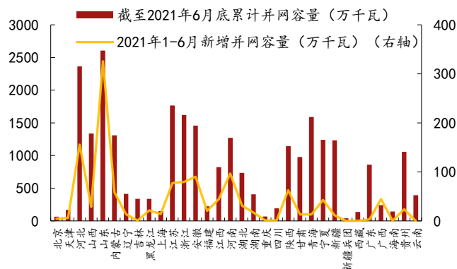
图 79: 2021 年上半年全国光伏发电建设全面开展
