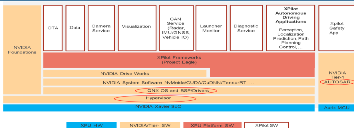
图表34： 小鹏域控制器软件框架
