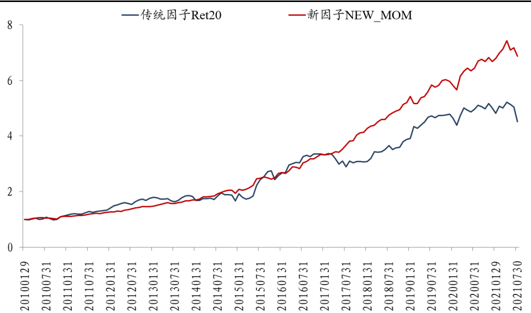
图 7: 新旧涨跌幅因子 5 分组多空对冲净值走势
