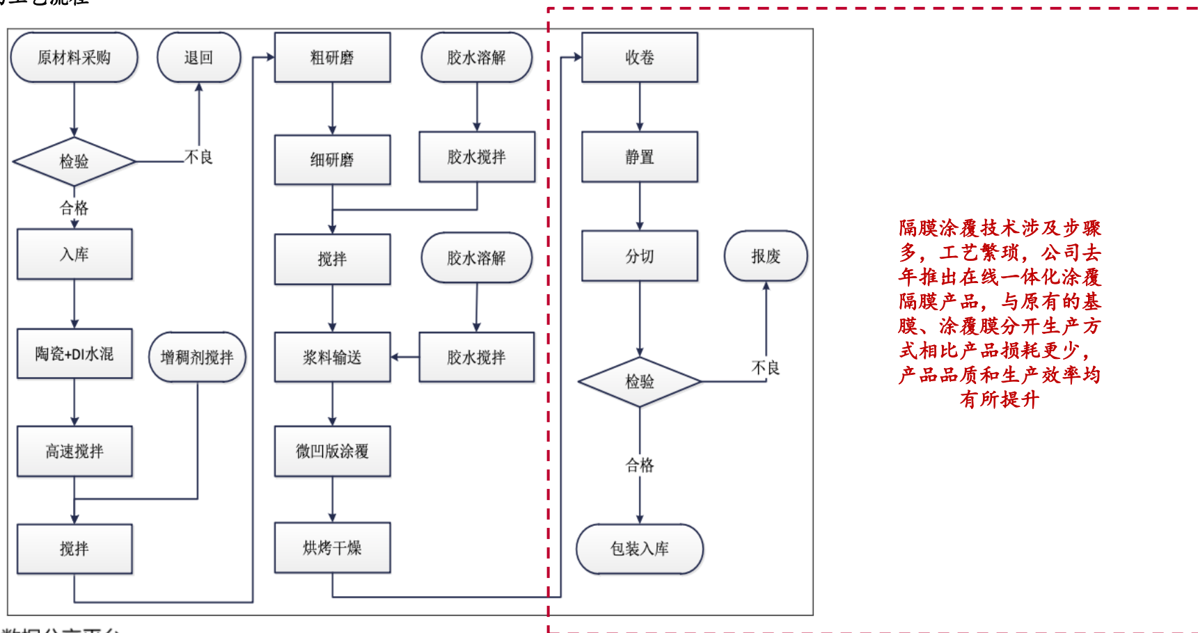
图表：涂覆隔膜的工艺流程
