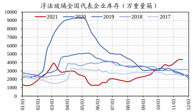
图 10：浮法玻璃库存周环比下滑 28 万重量箱
