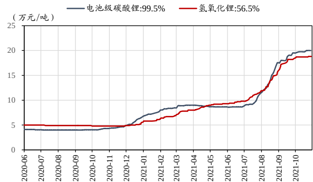
图 24: 碳酸锂/氢氧化锂价格周环比变化 0%/0.5%
