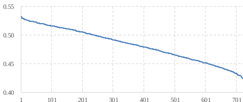
图 47：729 组回归拟合优度均值分布
