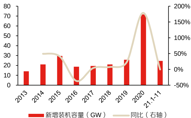
图 38：2020 年全国风力发电新增设备容量同比大增 178%
