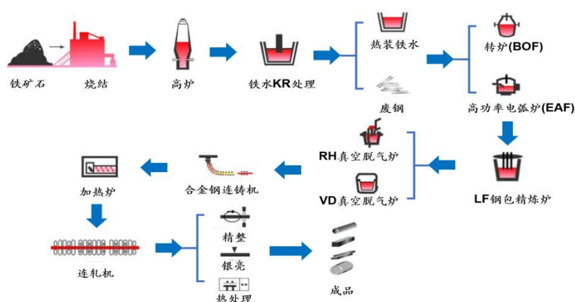
图 2：中信特钢主要产品生产工艺流程图
