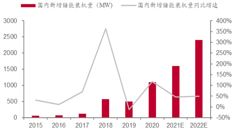
国内新增储能装机量高速增长
