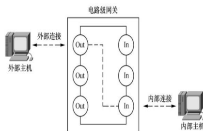
图 8、电路级网关防火墙
