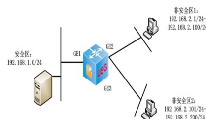
图 12、混合式防火墙
