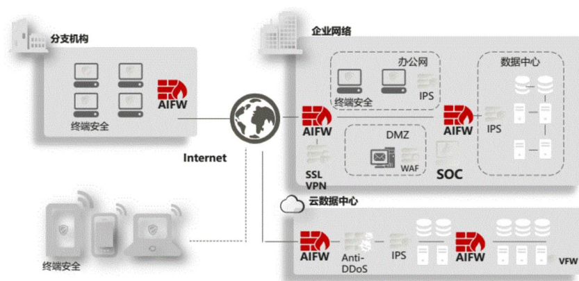
图 3、防火墙典型部署位置
