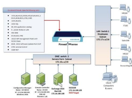
图 10、边界防火墙
