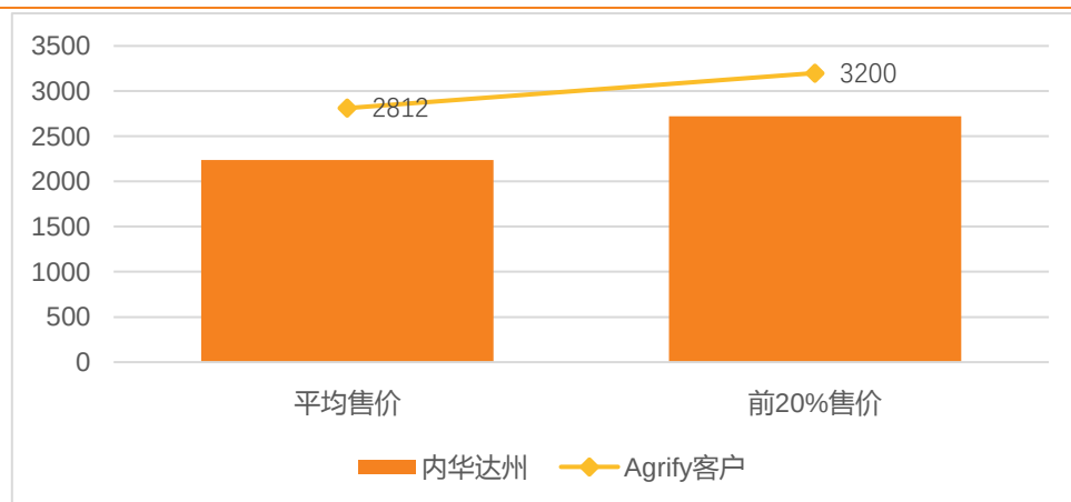
图 20: Agrify 与内华达州 cannabis 批发价对比 (美元/磅)
