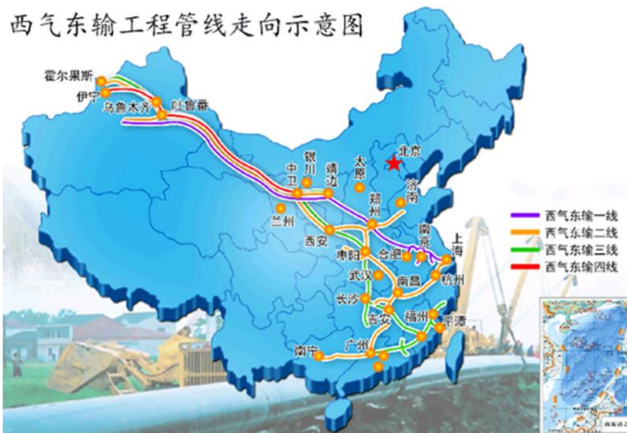
图 17: 西气东输工程管线走向示意图
