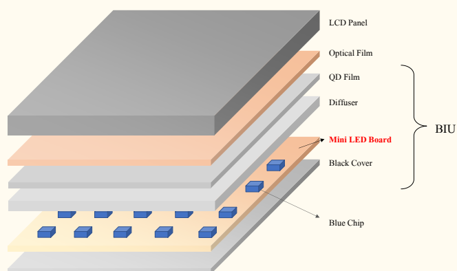
图表 51：Mini LED 用 PCB 板示意图
