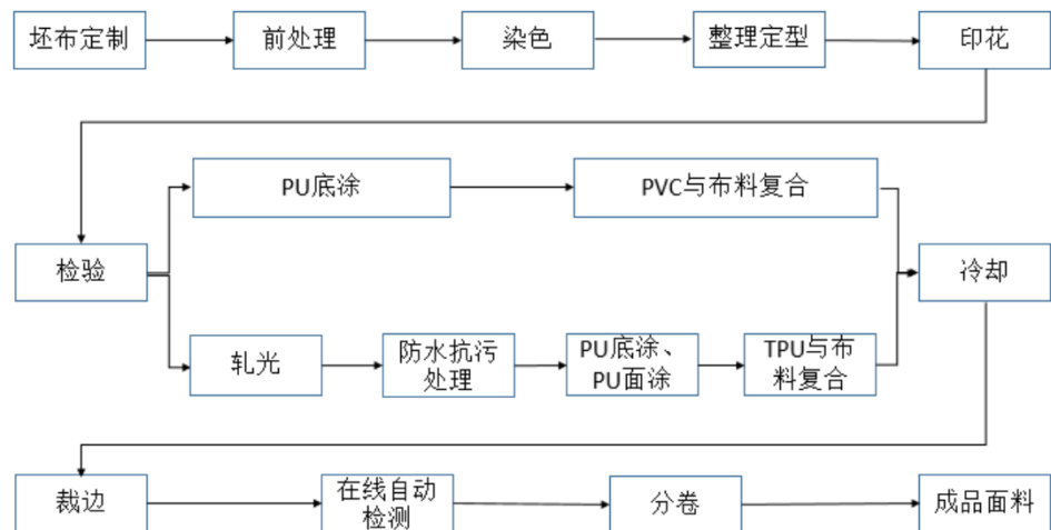
图 24: 一体化生产流程 (面料制作工艺)
