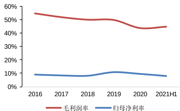
图 39：安克创新毛利率，归母净利率
