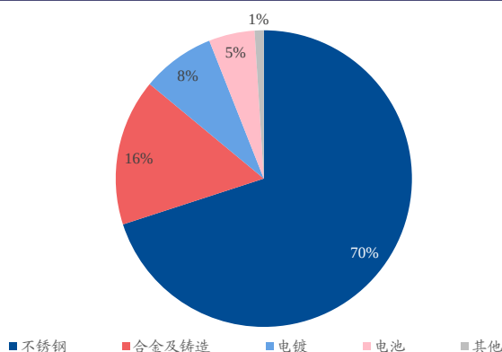
图 76、2019 年全球电池领域镍消费占比约 5%
