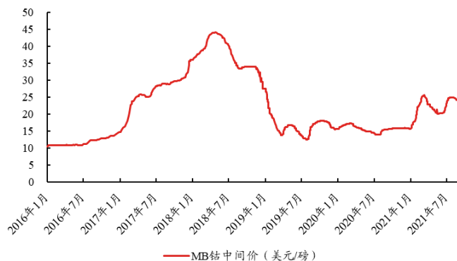
图 11、MB 钴价走势
