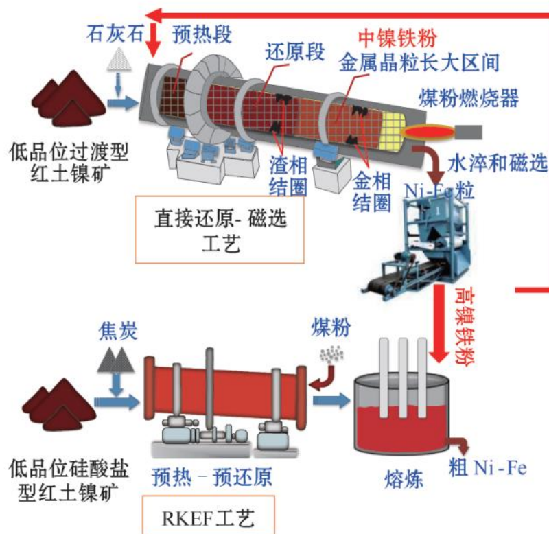
图 68、RKEF 工艺主要环节，在传统工艺基础上通过前端部分优化可拓展至低品位红土镍矿应用
