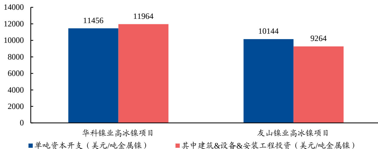
图 69、印尼投建 RKEF 生产线单吨资本开支预计约 11000-12000 美元/吨
