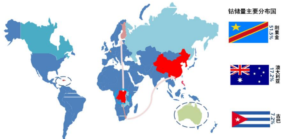
图 34、全球钴原料的流动，刚果金为主要产地，中国和芬兰是主要加工地
