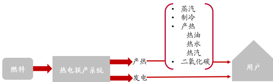
图表 31：热电联产示意图
