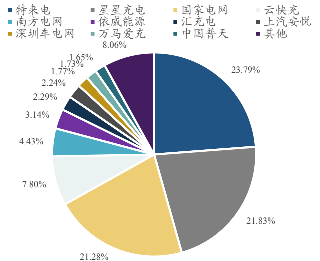
图 25: 2021 年 6 月中国各厂商公用充电桩占比 (%)
