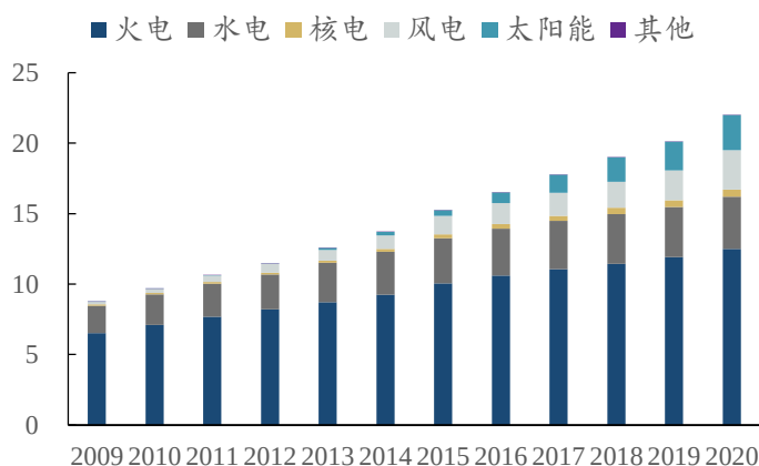
图 12：中国各类型发电装机容量（亿千瓦时）
